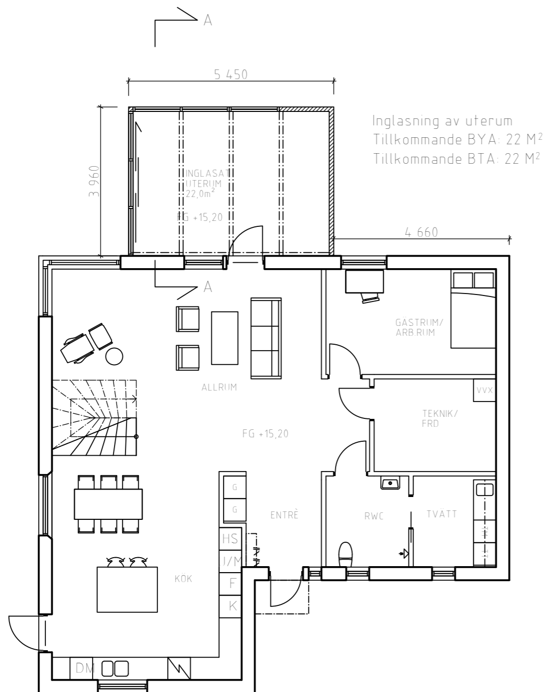
Plan 1, inglasat uterum
