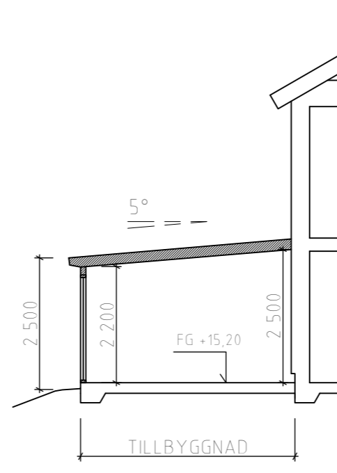
Sektion, inglasat uterum
